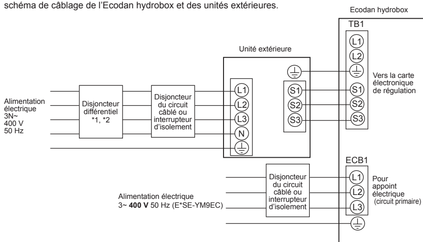
<Figure 4.4.3> Connexions électriques triphasées
